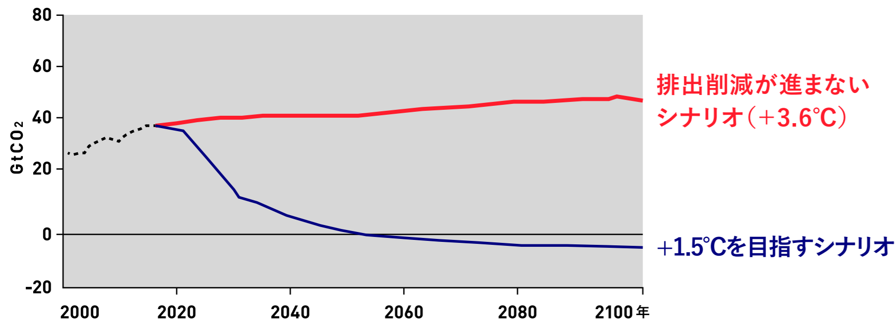
世界のCO 2 排出量の変化 IPCC「第6次評価報告書 第3作業部会」(2022)に基づき作成
