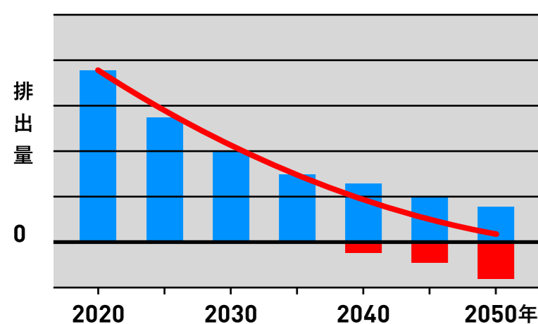
「実質ゼロ」への道筋のイメージ
